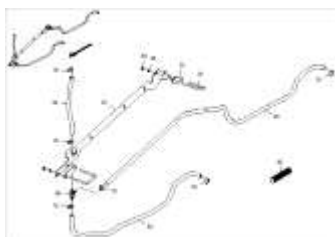
ЕТВ-0000011766, Распределительная шина 2 лемеха, междурядье 25 см с 01.2024
