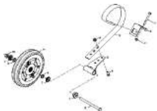
ЕТВ-0000003846, Монтажный комплект для катка выравнивателя 9001-2C (25,00 см) (2) с 02.2018
