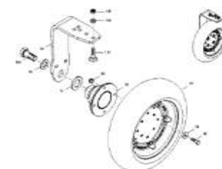
ЕТВ-0000005303, Задний каток ходовое колесо комплект дооснащения
