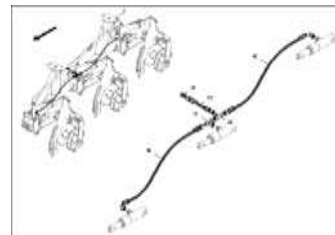
ЕТВ-0000010001, Монтажные части Гидравлический держатель сошников 3 сошника Расстояние между сошниками 25 см
