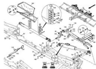
ЕТВ-0000011104, Primera DMC 9000 , Цилиндровая задняя поперечная рама Q1/2024
