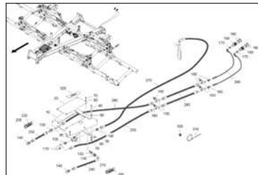
ETB-0000008380, Premiera DMC 9000-2C Super , базовая гидравлика
