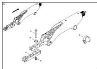
ЕТВ-0000009161, Переменная DMC с верхним звеном
