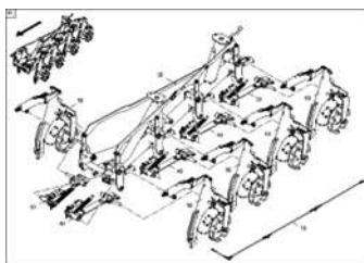
ЕТВ-0000009949, Держатель сошников 4 сошника правый, 1 левый
