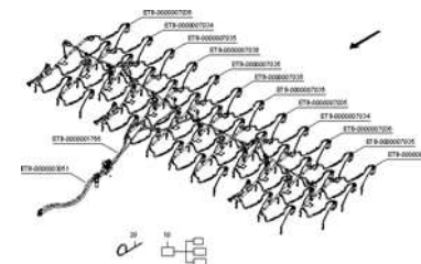
ЕТВ-0000003813, Набор насадок для жидких удобрений DMC 9000 XL-187.5
