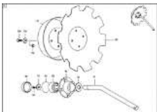
ЕТВ-0000005417, Дисковый трассировщик D 410 L 300
