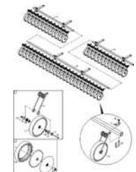
ЕТВ-0000003908, Монтажный комплект для катка выравнивателя на Primera DMC (18,75 см) (2) до 01.2018
