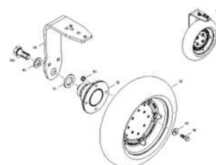
ЕТВ-0000005304, Задний каток, ходовое колесо
