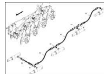
ЕТВ-0000009955, Монтажные детали гидравлического держателя лопастей 4 правых, 1 левых
