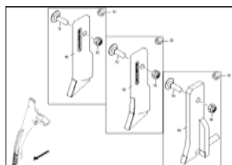
ЕТВ-0000003799, Долотовидный сошник
