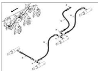
ЕТВ-0000009994, Монтажные части гидравлический держатель сошников 3 правый, 1 левый
