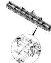
ЕТВ-0000003836, Монтажный комплект для катка- выравнивателя на Primera DMC (25 см) (1) до 01.2018
