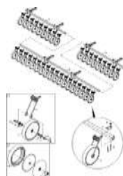
ЕТВ-0000003837, Монтажный комплект для катка- выравнивателя на Primera DMC (25 см) (2) до 01.2018
