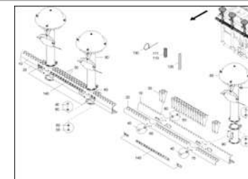
ЕТВ-0000005352, Распределение семян и удобрений DMC 9 м, междурядья 25 см с технологической колеей
