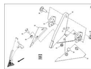
ЕТВ-0000008932, Набор долот для гусиной лапки 200 с бронированной пластиной
