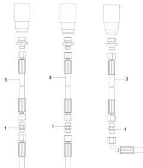
Verlängerung der Schläuche zum Striegel und zur Vorauslaufmarkierung
