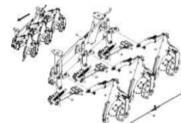
ЕТВ-0000009877, Держатель сошников 3 сошника
