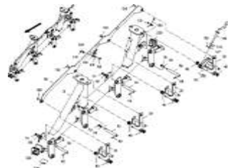
ЕТВ-0000009874, Держатель сошников 4 сошника
