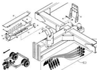
ETB-0000005654, Передняя тележка DMC (2)
