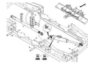
ЕТВ-0000011106, Primera DMC 9000 , Передний цилиндр поперечной рамы Q1/2024
