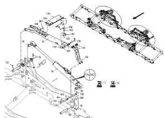
ETB-0000008332, Primera DMC 9000-2C Super , Поперечная рама (8)
