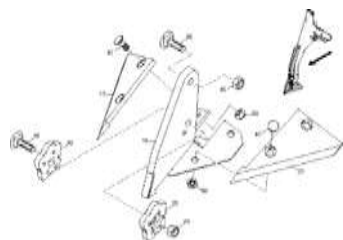
ЕТВ-0000003801, Долотовидный сошник для ленточного посева 200
