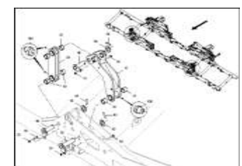
ETB-0000008344, Primera DMC 9000-2C Super, Поперечная рама (5)
