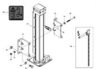
ETB-0000005655, Опорная стойка регулируемая DMC
