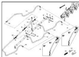
ЕТВ-0000007035, Набор навесного оборудования для жидких удобрений 4 сошника 187,5
