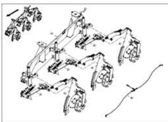
ЕТВ-0000009995, Держатель сошников 3 сошника 25 см расстояние между сошниками
