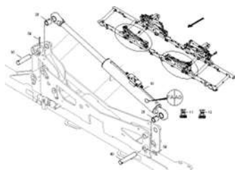
ETB-0000008336, Primera DMC 9000-2C Super , Поперечная рама (7)
