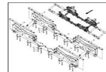
ETB-0000008370, Primera DMC 9000-2C Super, Поперечная рама (2)
