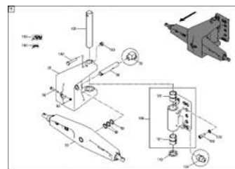
ЕТВ-0000008610, Нижняя тяга сцепки Cat. 4H
