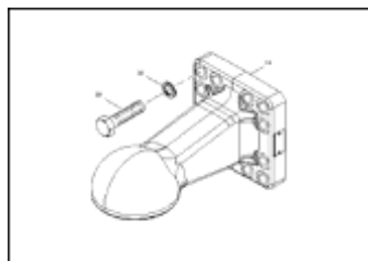
ЕТВ-0000008622, Тяговая шаровая муфта K110 6T
