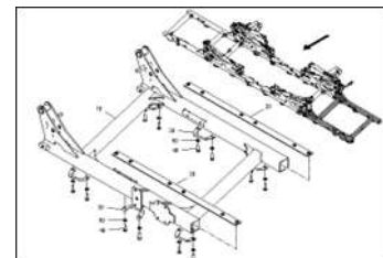
ETB-0000008372, Primera DMC 9000-2C Super, Поперечная рама (1)
