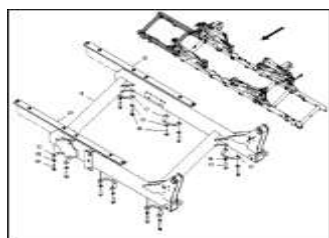
ETB-0000008369, Primera DMC 9000-2C Super, Поперечная рама (3)
