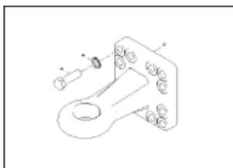
ЕТВ-0000008631, Буксировочная проушина D=58 (9000-2C Super)
