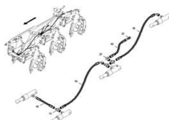
ЕТВ-0000010016, Монтажные части гидравлический держатель сошников 3 сошника правый, 1 левый расстояние между сошниками 25 см
