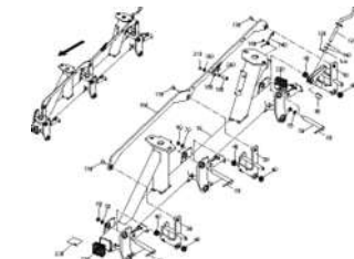
ЕТВ-0000010026, Держатель сошников 3 сошника 25 см расстояние между сошниками
