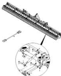
ЕТВ-0000003907, Монтажный комплект для катка выравнивателя на Primera DMC (18,75 см) (1) до 01.2018
