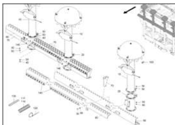
ЕТВ-0000006564, Распределение семян и удобрений DMC 9 м, междурядья 18,75 см с технологической колеей
