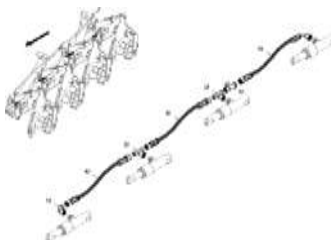
ЕТВ-0000009944, Монтажные части гидравлического держателя сошников 4 сошника
