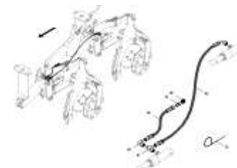
ЕТВ-0000010030, Монтажные части Гидравлический держатель сошников 3 сошника Расстояние между сошниками 25 см
