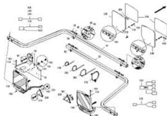
ЕТВ-0000005767, Освещение DMC 4,5 м длинн.
