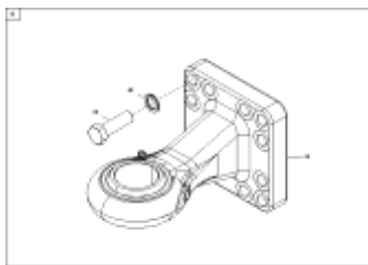
ЕТВ-0000008651, Тянущая проушина D=71 (шаровая опора)
