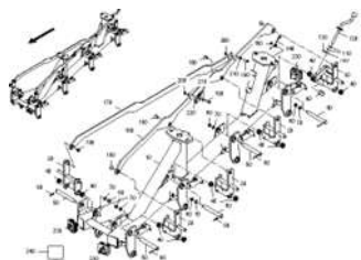
ЕТВ-0000009793, Держатель сошников 4 сошника правый, 1 левый (1)
