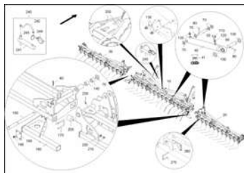
ЕТВ-0000003828, Выравниватель Exakt 15 мм для Primera DMC 9 м Super / XL (2) до 01.2018
