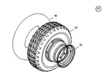
ETB-0000005656, Колесо в сборе 11.5/80
