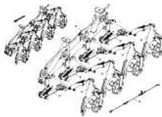
ЕТВ-0000009860, Держатель сошников 4 сошника
