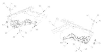
ЕТВ-6000000002, Консоли
