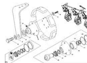
ЕТВ-0000005923, Узел держателя катка со скобами
