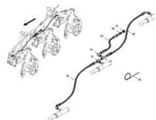
ЕТВ-0000010025, Монтажные части Гидравлический держатель сошников 3 сошника Расстояние между сошниками 25 см
