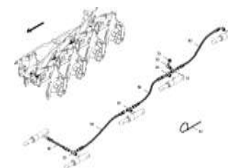
ЕТВ-0000009841, Монтажные детали гидравлического держателя лопастей 4 правых, 1 левых
