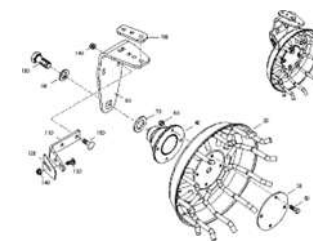
ЕТВ-0000005301, Каток для каменистой почвы (111800)
