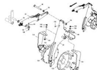
ЕТВ-0000009889, Монтажные детали, верхняя тяга, лемех, левое посадочное место для железной катушки
