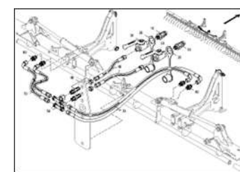
ЕТВ-0000003834, Выравниватель Exakt DMC 9 м XL/ гидравлические разъемы рама выравнивателя
