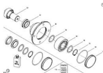
ЕТВ-0000005302, Подшипниковый узел
