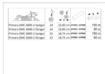
ЕТВ-0000006135, Комплекты шлангов Primera DMC
