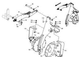
ЕТВ-0000009889, Монтажные детали, верхняя тяга, лемех, левое посадочное место для железной катушки
