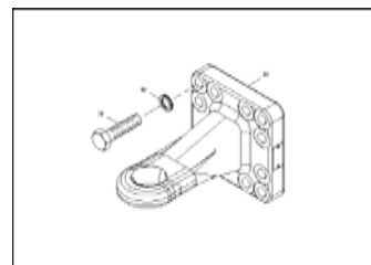
ЕТВ-0000008625, Буксировочная проушина 160x160 M20/ D46 (9000-2C Super)
