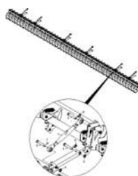
ЕТВ-0000003849, Комплект каток-выравниватель DMC 9M Super/XL 250 (1) до 01.2018
