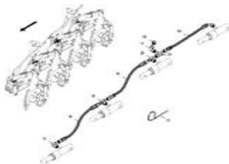
ЕТВ-0000009875, Монтажные детали гидравлики 4 сошника
