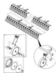
ЕТВ-0000003850, Комплект каток-выравниватель DMC 9M Super/XL 250 (2) до 01.2018
