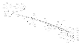
ЕТВ-6000000003, Стрела
