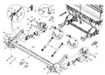
ETB-0000005089, Задняя навесная система 6000L/13000L
