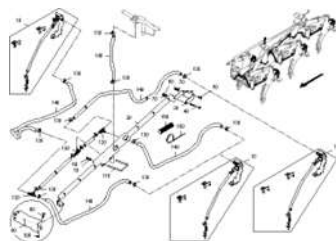
ЕТВ-0000003824, Монтажный комплект для жидкого удобрения 4 сош. 250
