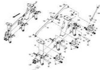
ЕТВ-0000009879, Держатель сошников 3 сошника
