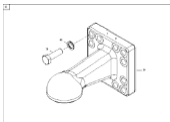
ЕТВ-0000008620, Тяговая шаровая муфта M20/K80
