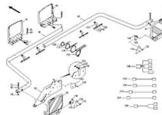
ЕТВ-0000000395, Освещение DMC 4,5 м длинн.
