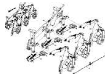
ЕТВ-0000009877, Держатель сошников 3 сошника
