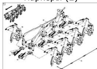
ЕТВ-0000009949, Держатель сошников 4 сошника правый, 1 левый
