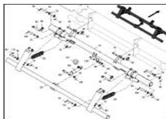
ЕТВ-0000009150, Роликовая борона DMC - правая рама ролика 2,1 м
