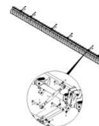
ЕТВ-0000003840, Комплект каток-выравниватель DMC 9M Super/XL (1) до 01.2018
